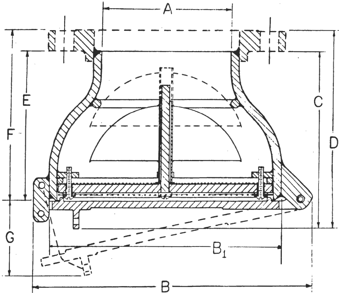
Dimensions -- Inches
